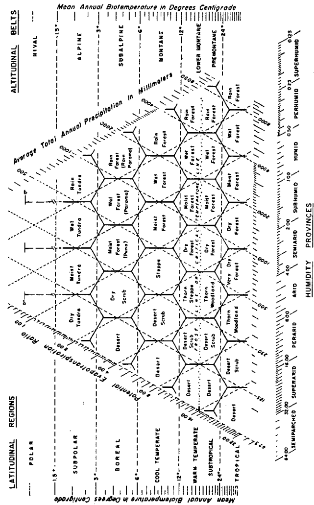
Abb. 2.1.i: HOLDRIDGE's Klassifikation der Lebenszonen (Life-zones) bzw. der Pflanzenformationen (HOLDRIDGE, 1967)
